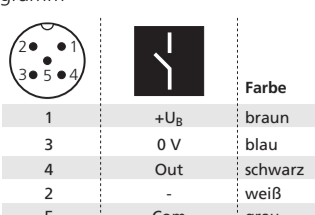
Abb. 1: Pin-Belegung mit Sicht auf den Sensor-Stecker und Farb-Kodierung der Balluff-Anschlusskabel
