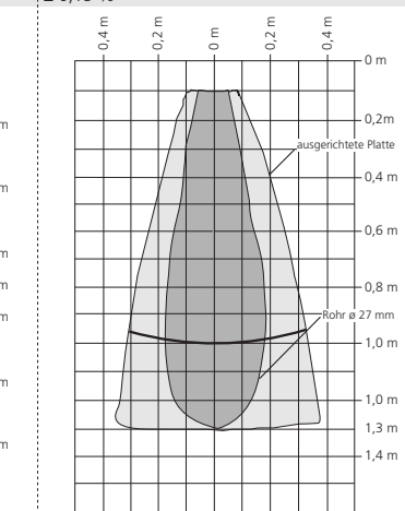
Abb. 3: Einstellung des Schaltpunktes bei unterschiedlicher Bewegungsrichtung des Objekts
