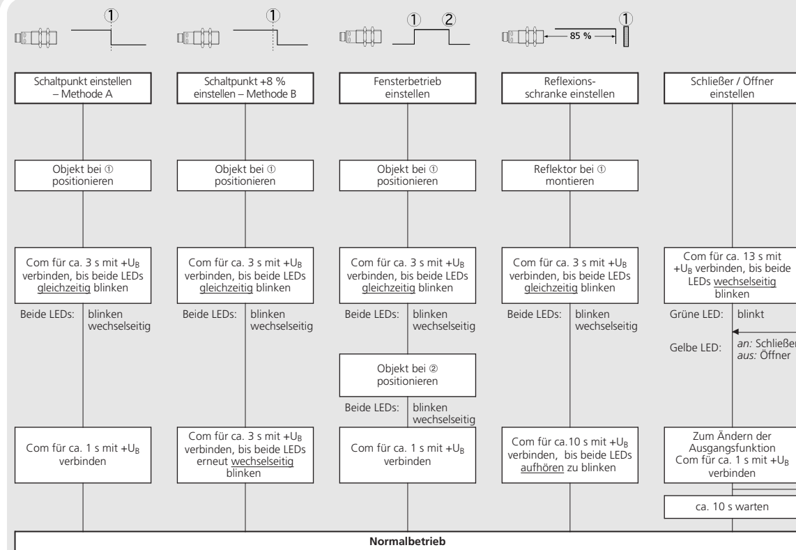
Schaltausgang einstellen
