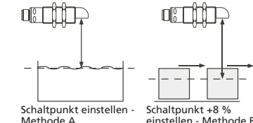
Abb. 3: Einstellung des Schaltpunktes bei unterschiedlicher Bewegungsrichtung des Objekts
