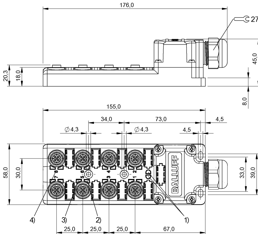
1) Индик. раб. зел. потенциал 2) СД ЖЛТ для S2 на конт. 2 3) СД ЖЛТ для S1 на конт. 2 4) Нумерация гнезд
