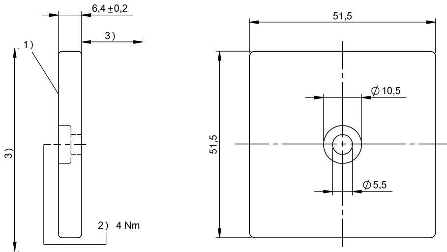
1) Активная поверхность 2) Момент затяжки 3) см. таблицу Головка S/L
