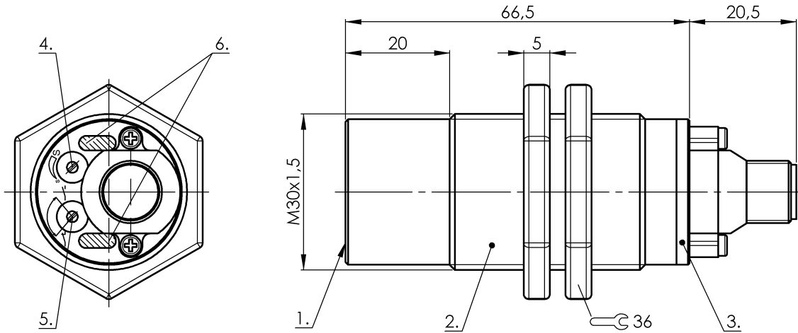
1) Активная поверхность 2) Корпус 3) Крышка 4) Потенциометр 5) По выбору замыкатель или размыкатель 6) Функциональный СД
