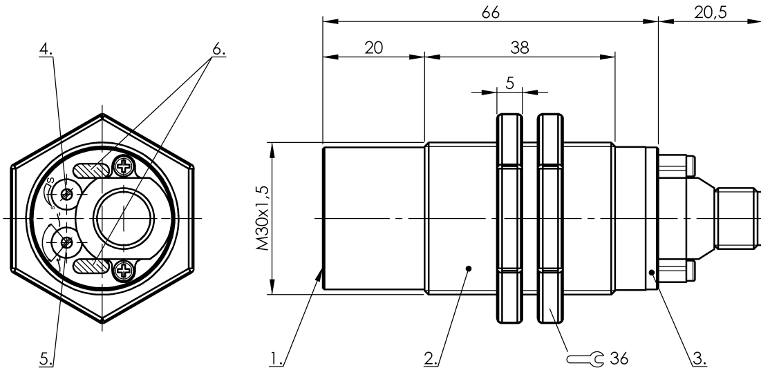
1) Активная поверхность 2) Корпус 3) Крышка 4) Потенциометр 5) По выбору замыкатель или размыкатель 6) Функциональный СД
