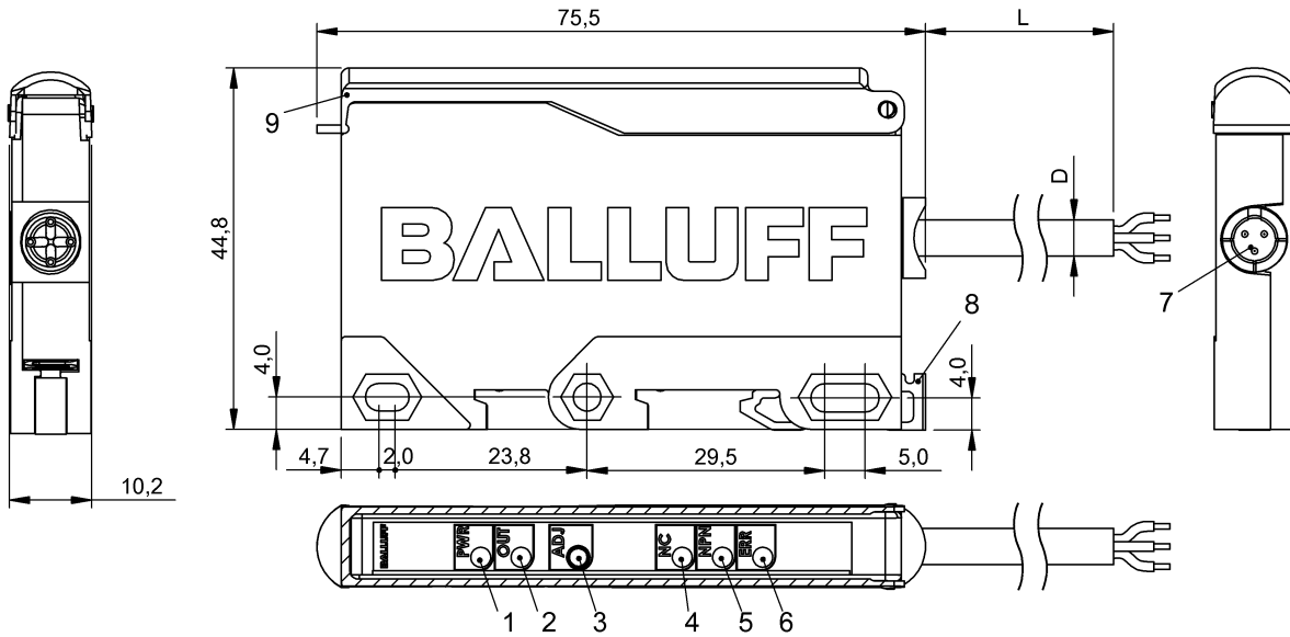
1) СД напряжения питания 2) Функциональный СД 3) Sn 4) СД функ. размыкателя активен 5) СД ступени переключения N-P-N акт. 6) СД - сбой 7) Штекерный разъем датчика 8) Монтаж защитной шины 35 мм 9) Заслонка
